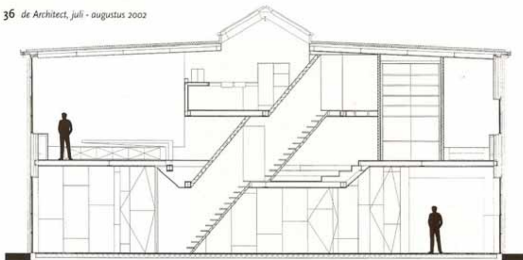
Doorsnede
